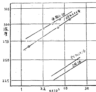
第11圖 K \times 10^3 の温度による変化
