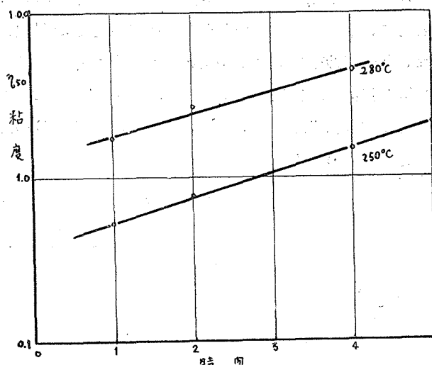
第3圖 No.1 鳥賊原油加熱處理の粘度變化
