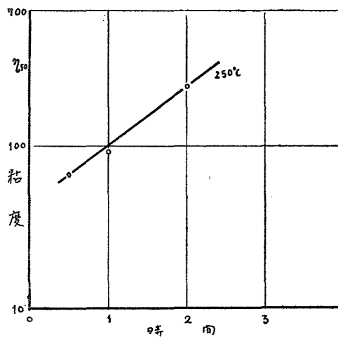
第 8 圖 No. 6 の Bodying 中の粘度変化
