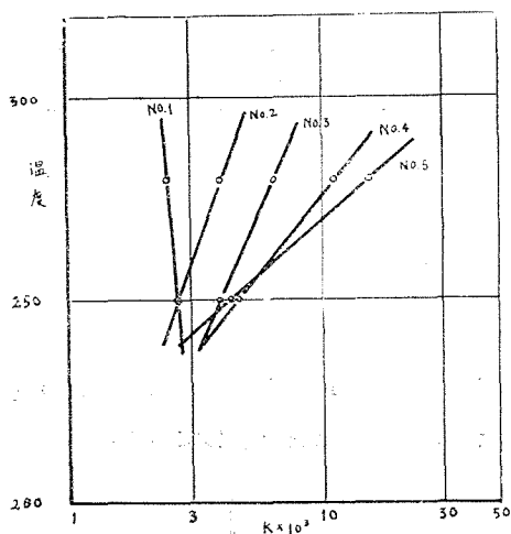
第10圖 K \times 10^3 の温度による変化
