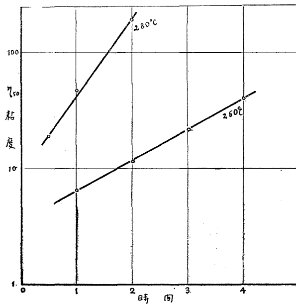
第 6 圖 No. 4 の Bodying 中の粘度変化
