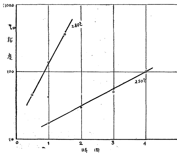
第 7 圖 No. 5 の Bodying 中の粘度変化
