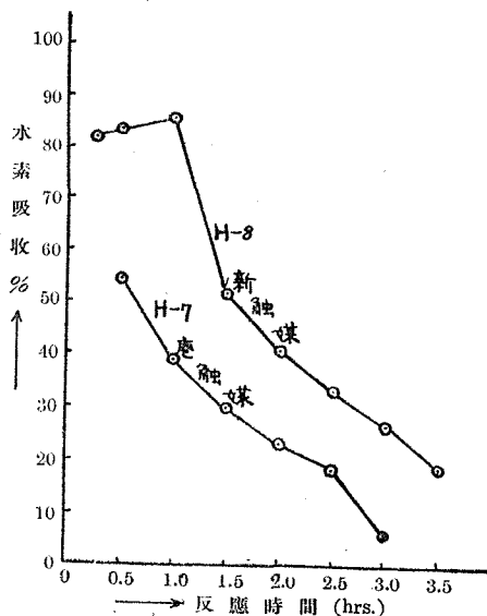
第3圖 新觸媒と廢觸媒の活性の比較 (Ni+Co=1.0%)
