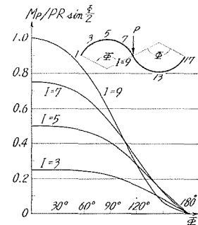
図-7 図の荷重状態における各点曲げモーメントと中心角 \phi の関係
