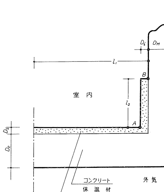
図-3-4 断面形
