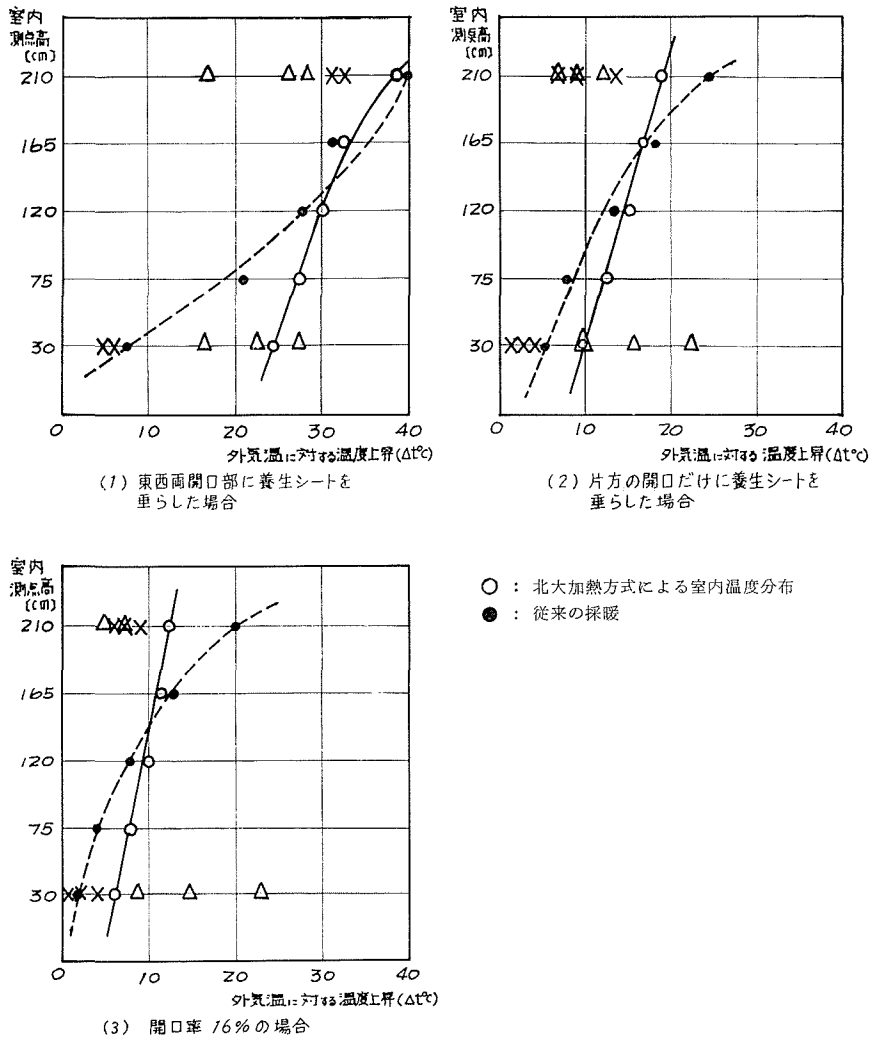
図-5 北大加熱方式と従来採暖方法における温度分布比較
