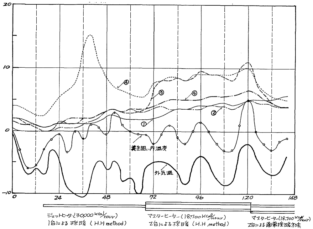
図-16 現場実験 (その2) グラウトペースト温度分布
