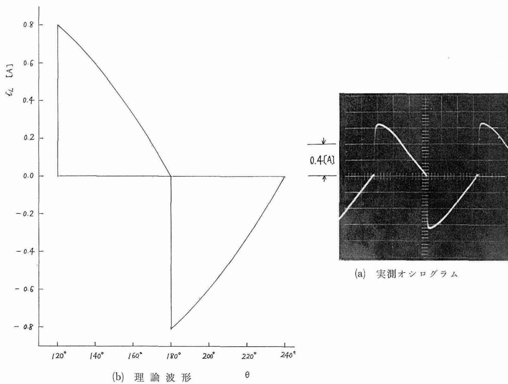
第10図 R=50[\Omega] , X=0 , \alpha=\alpha_c の場合の負荷電流波形 ( V=42.4 volt)
