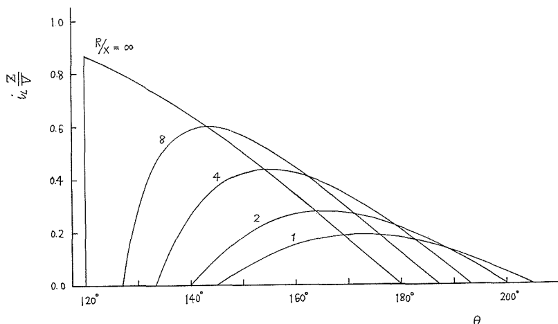
第6図 R/X による負荷電流波形の変化
