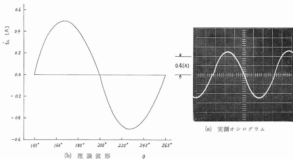
第 7 図 R/X=1 , \alpha=\alpha_c の場合の負荷電流波形 ( V=56.6 volt)
