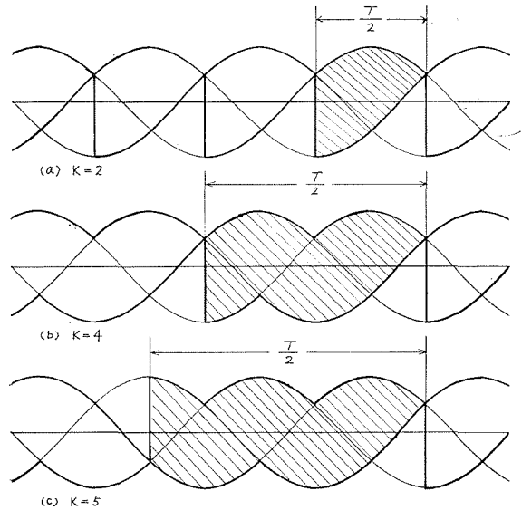
第 1 図 K=2, 4, 5 の場合の負荷電圧波形 ( \alpha=0 のとき)
