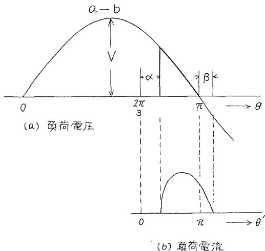
第 4 図 負荷電圧と負荷電流との関係
