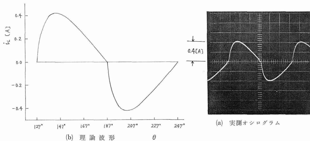
第9図 R/X=8 , \alpha=\alpha_c の場合の負荷電流波形 ( V=84.8 volt)
