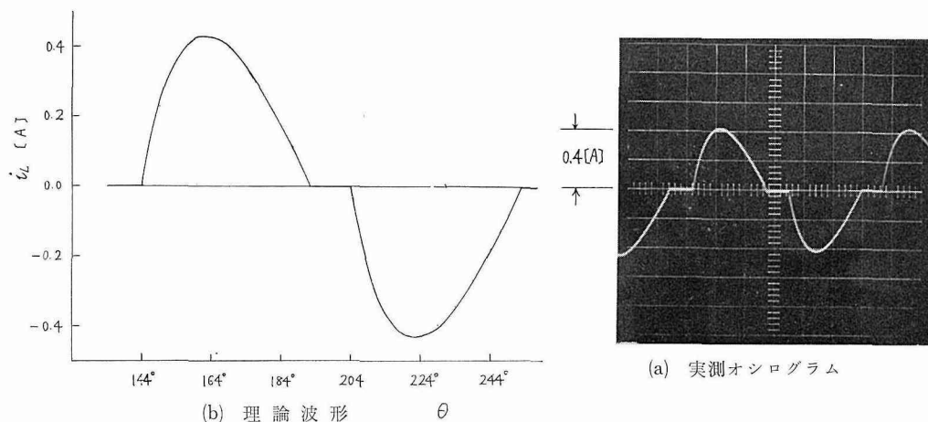
第 11 図 R/X=1 , \alpha=24^\circ の場合の負荷電流波形 ( V=84.8 volt)
