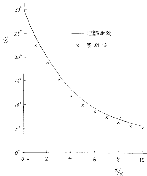
第5図 臨界制御角 \alpha_c と R/X との関係
