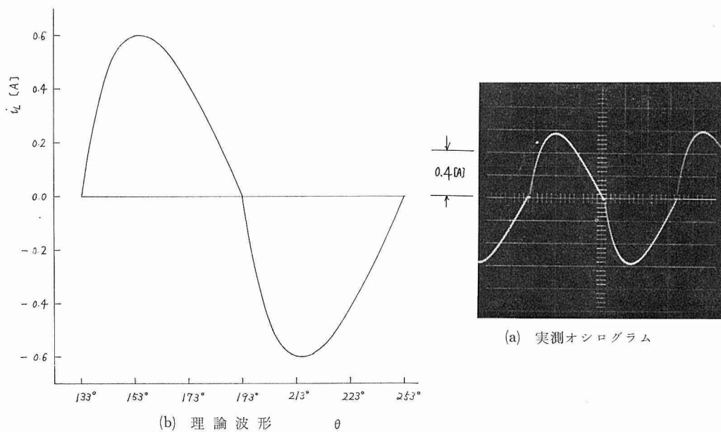
第 8 図 R/X=4 , \alpha=\alpha_c の場合の負荷電流波形 ( V=84.8 volt)
