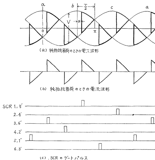
第 3 図 負荷電圧及び電流と SCR のゲートパルス位置との関係
