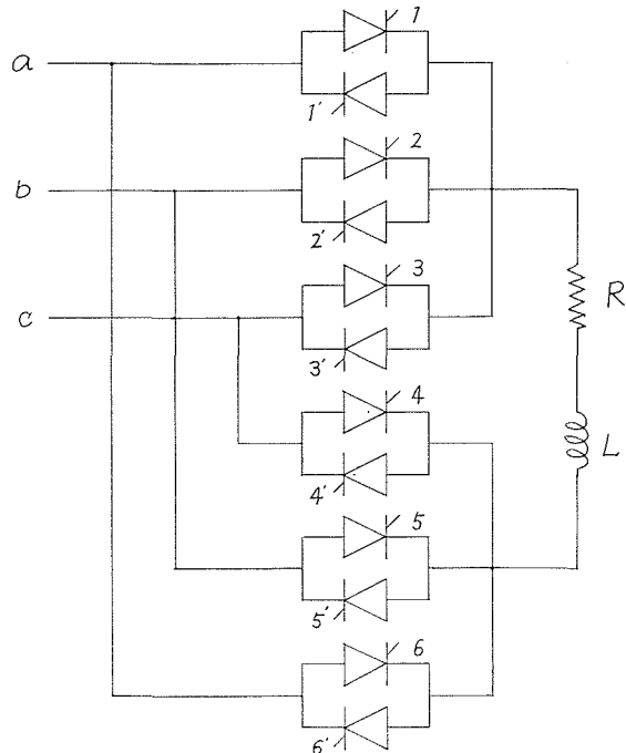
第 2 図 定比式 SCR 周波数変換器
