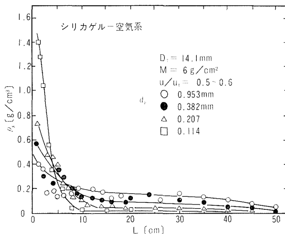
図 24 整流板からの高さ粒子密度（粒径の影響）
