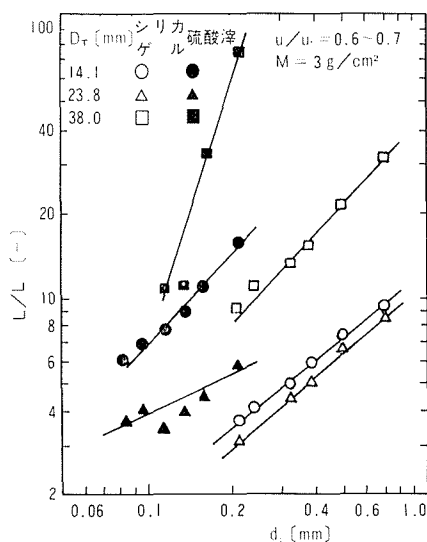
図10 粒径と層高
