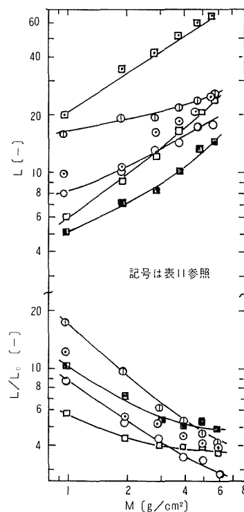
図11 浮遊量と層高
