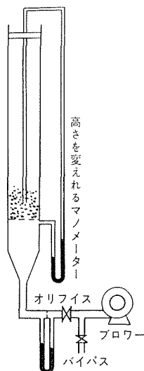
図 23 粒子密度測定装置
