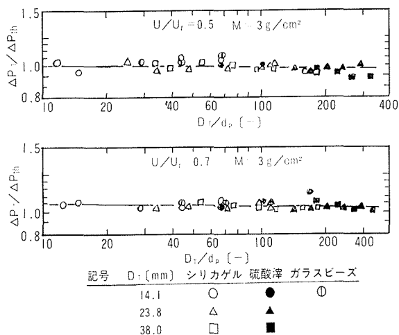
図 21 塔径粒径比と圧力損失比
