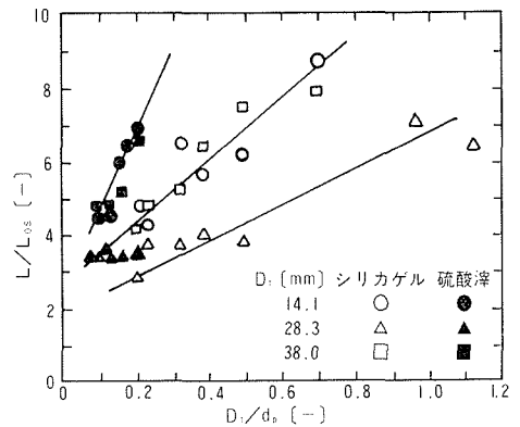
図 13 粒径と層高
