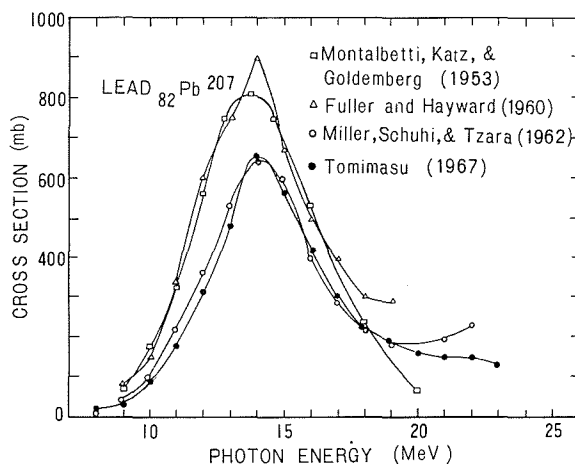
第5図 (r, n) 反応の巨大共鳴の例、鉛のデータ (文献14) より)
