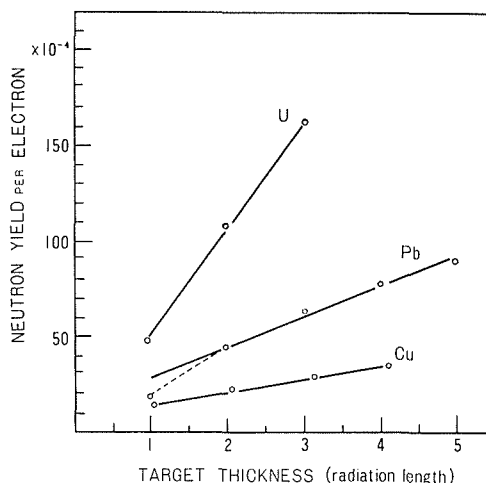
第 9 図 中性子収量のターゲット厚さ依存性 (実験値) 16) 4 放射長までは、ほぼ直線的に増加する。
