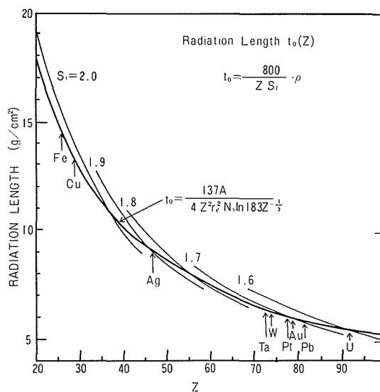
第1図 (4) 式による放射長の計算値と通常の計算式
