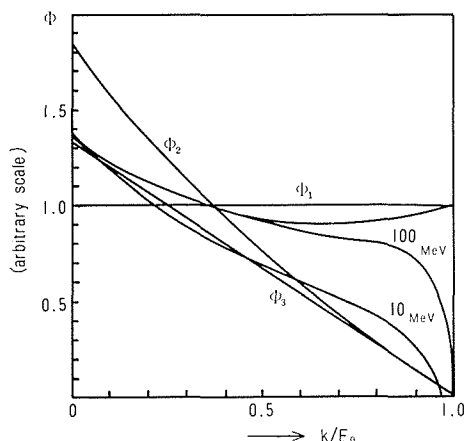
第3図 制動放射の近似スペクトルの比較 太線は薄いターゲットの計算 細線 \phi_1 : 一定スペクトル \phi_2 : \ln\{(1+a_1)/(k/E_0+a_1)\} \phi_3 : a_2(1-k/E_0) a_1, a_2 は定数
