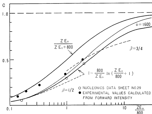
第2図 制動放射の電子-光子エネルギー変換効率
