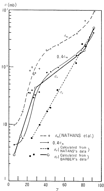
第6図 巨大共鳴積分 \sigma_r を実験値から計算した値 \sigma_r = 0.4\sigma_m とする BARBER と GEORGE との実験値とよく一致する
