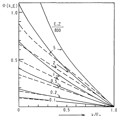
第4図 厚いターゲットの制動放射の近似スペクトル 実線は (12) 式 破線は (12a) 式で \beta=1/2
