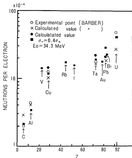
第 8 図 中性子収量の原子番号依存性 白丸は BARBER による実験値 ×印は BARBER らの計算値 黒丸はここで述べた方法で実験値にできるだけ一致させるようにした \sigma_r を利用した場合 ■印は \sigma_r=0.4\sigma_m とした場合の計算値
