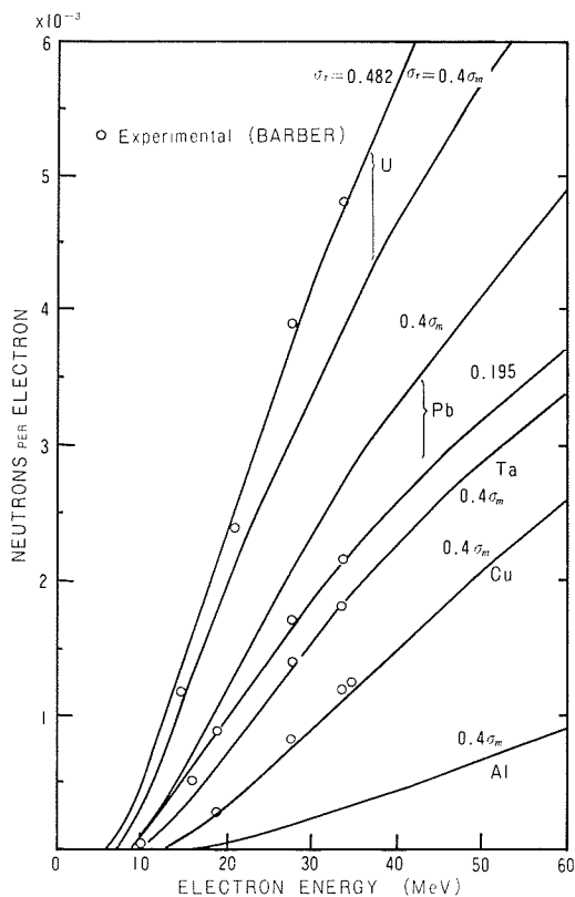
第7図 入射電子エネルギーによる中性子収量の変化の計算と実験値
