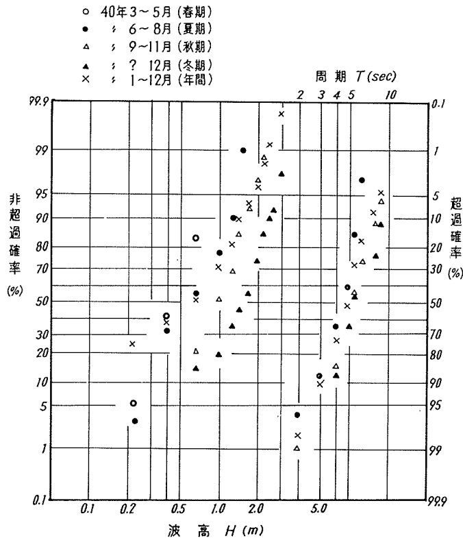
図-9 紋別港波高、周期の超過確率
