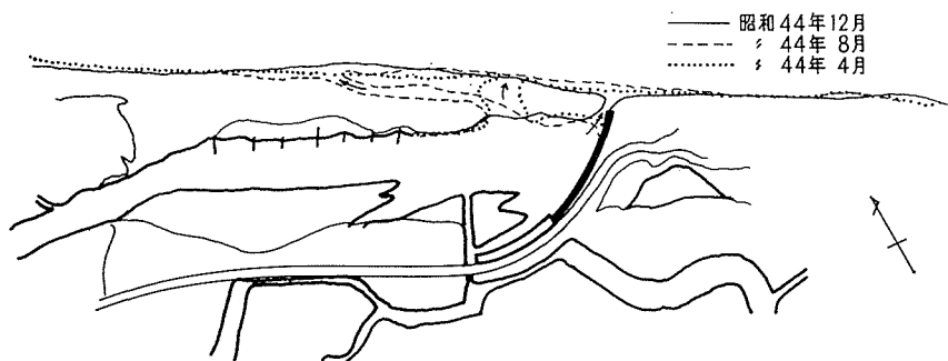
図-12 昭和44年4月、8月、12月の滑川河口
