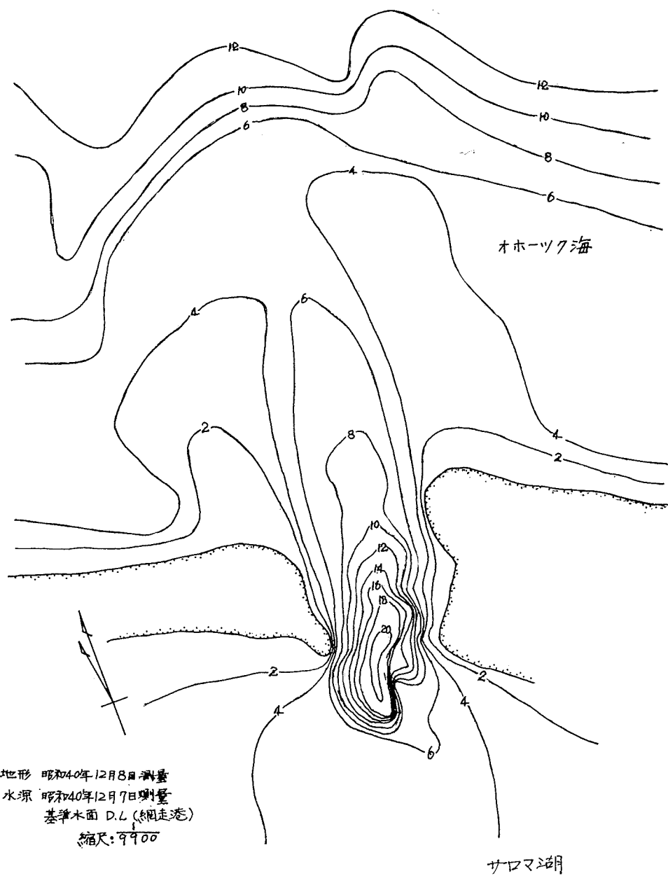
図—5 サロマ湖口深浅測量図 (昭和40年12月7日測量)
