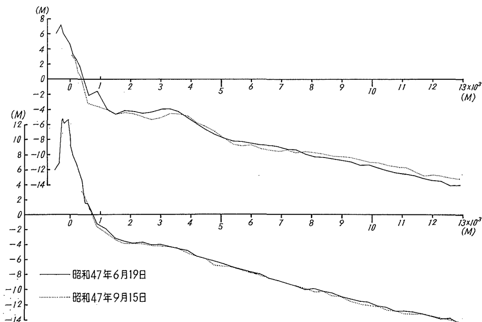
図-10 サロマ湖前面のオホーツク海海底地形の例
