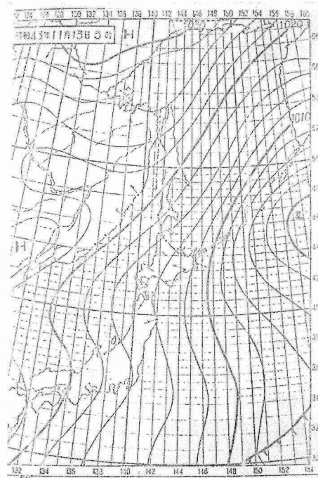
図—14c 昭和43年11月13日03時天気図
