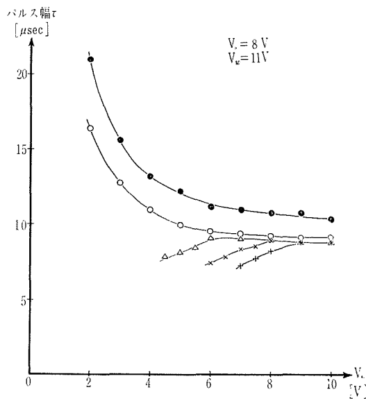
図 6 書き込み特性 (II)
