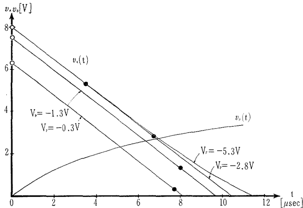
図8 v_A(t) および v_B(t) の計算値
