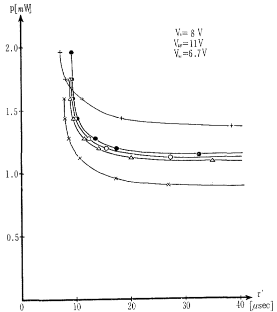
図10 消費電力 (II)
