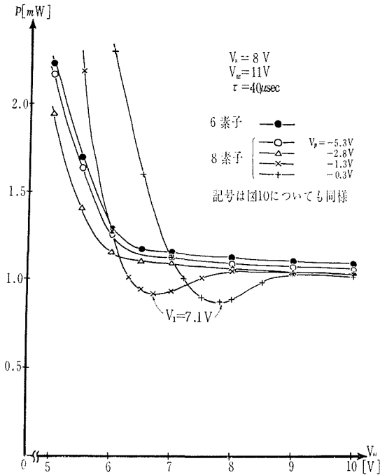
図9 消費電力 (I)
