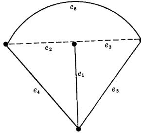
図 2-2 例題 2-1 のグラフ Fig. 2-2 A hybrid graph of example 2-1
