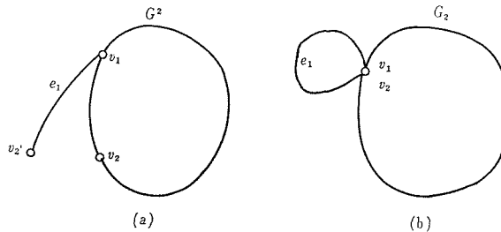
図 3-1 補題 9 の説明のためのグラフ
