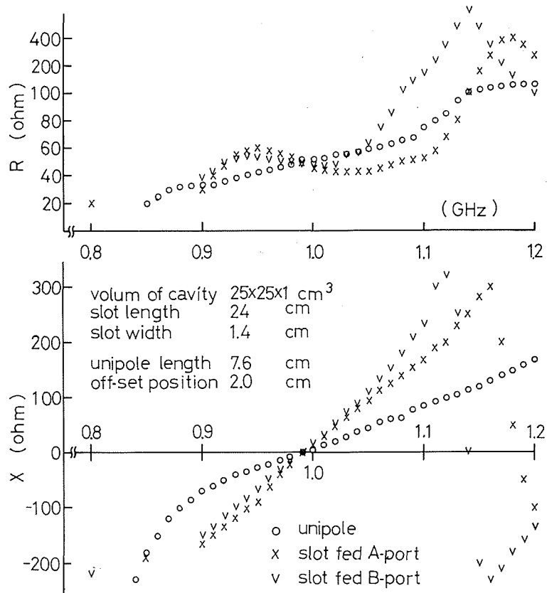
Fig. 7 Input impedance
