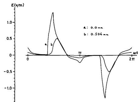
図16 異った深さでの電界の強さの波形
