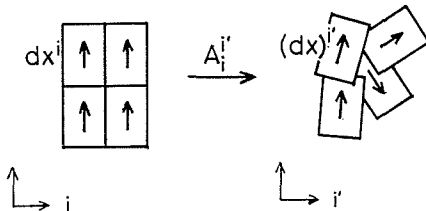
第1図 物理空間から視空間への変換
