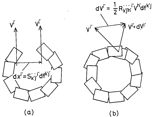
第3図 (a) 振率と (b) 曲率
