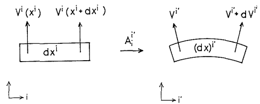
第2図 擬平行性
