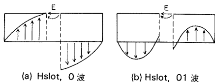
図6 薄型空胴スロットアンテナ上に励振される漏洩波 H_{slot,0} 波と H_{slot,01} 波の電界分布
