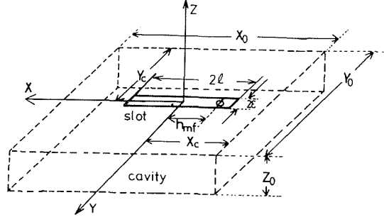
図3 空胴付スロットアンテナ
