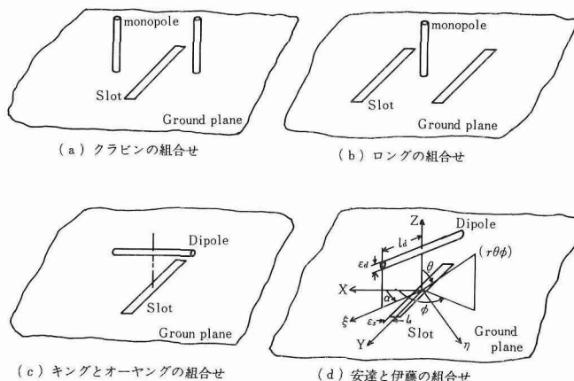
図10 スロットと線状アンテナの各種組合せ
