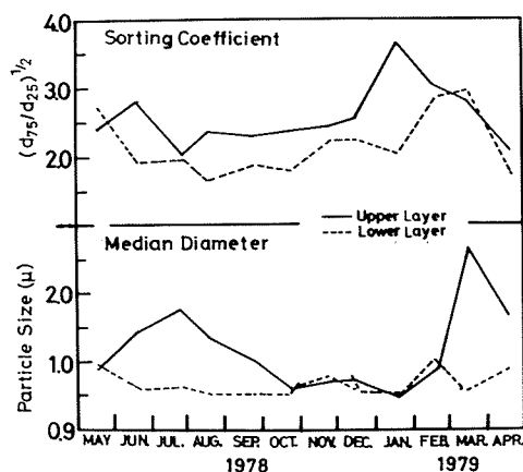
図-14 中央粒径、篩い分け係数の年変化
