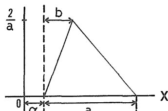
図7 三角分布
