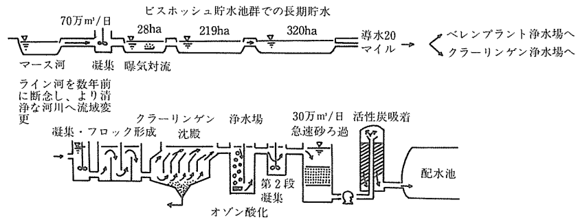
図-4 ロッテルダム水道マース・ビスボッシュ・クラールンゲン系の処理フロー
