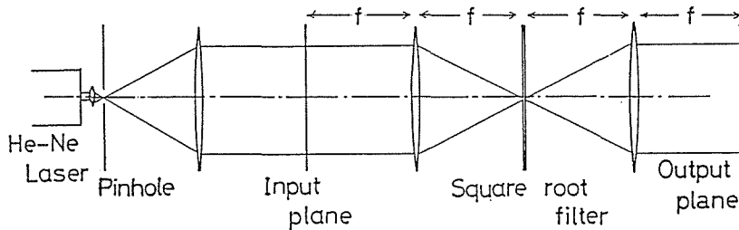
図1 コヒーレント光再回折空間フィルタリング系
