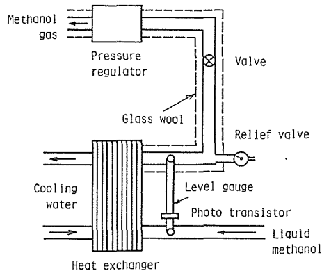
図2 メタノールガス発生装置(改良タイプ)
