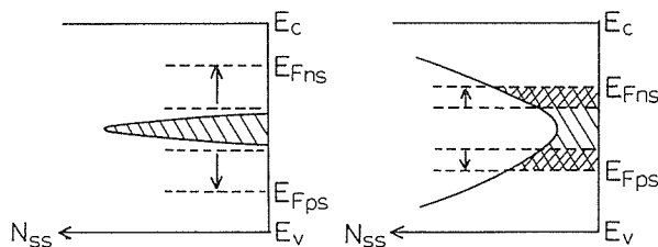
図5(b) 擬フェルミ準位の分離
