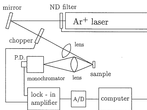
図6 測定系
