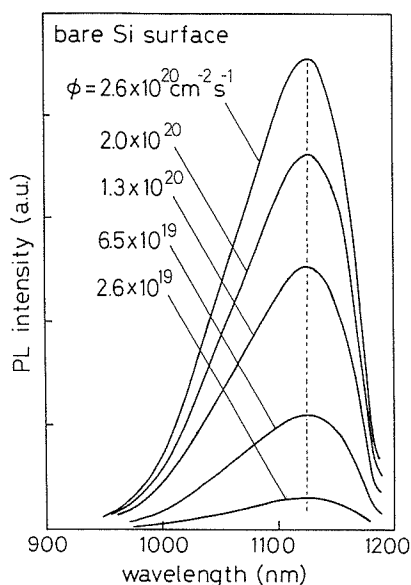
図7 PL のスペクトル形状
