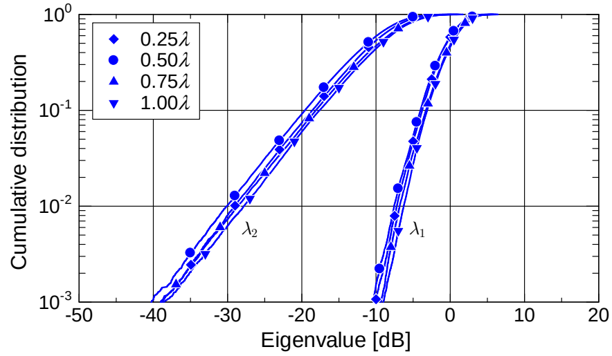
(a) TX-x/RX-x
