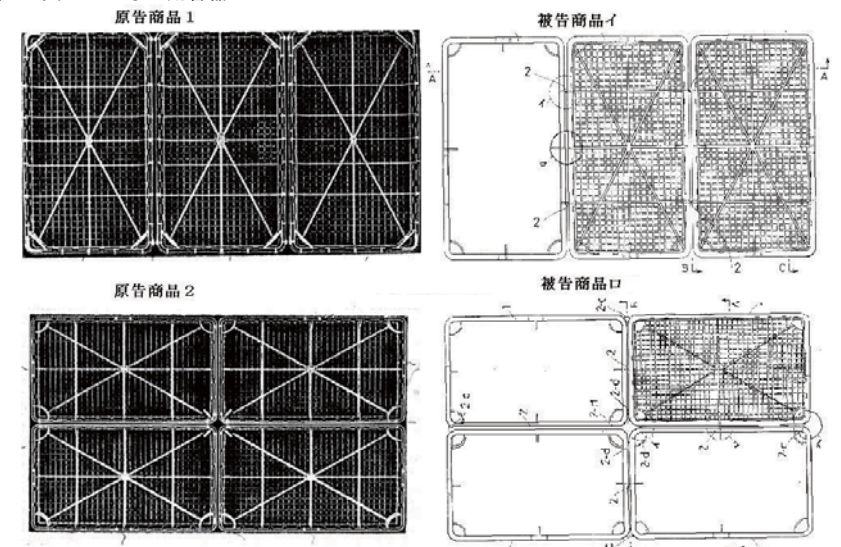
第41図 いかなご用容器
