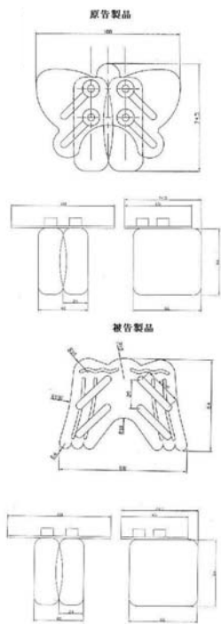
第35図 磁気活水器
