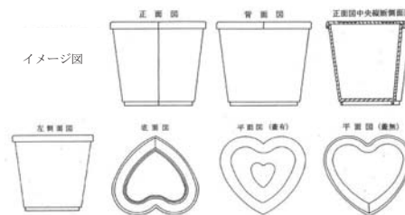
第6図 ハート型包装容器
