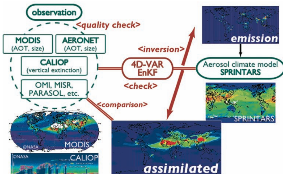
図3：SPRINTARS へのデータ同化手法適用の概念図。
