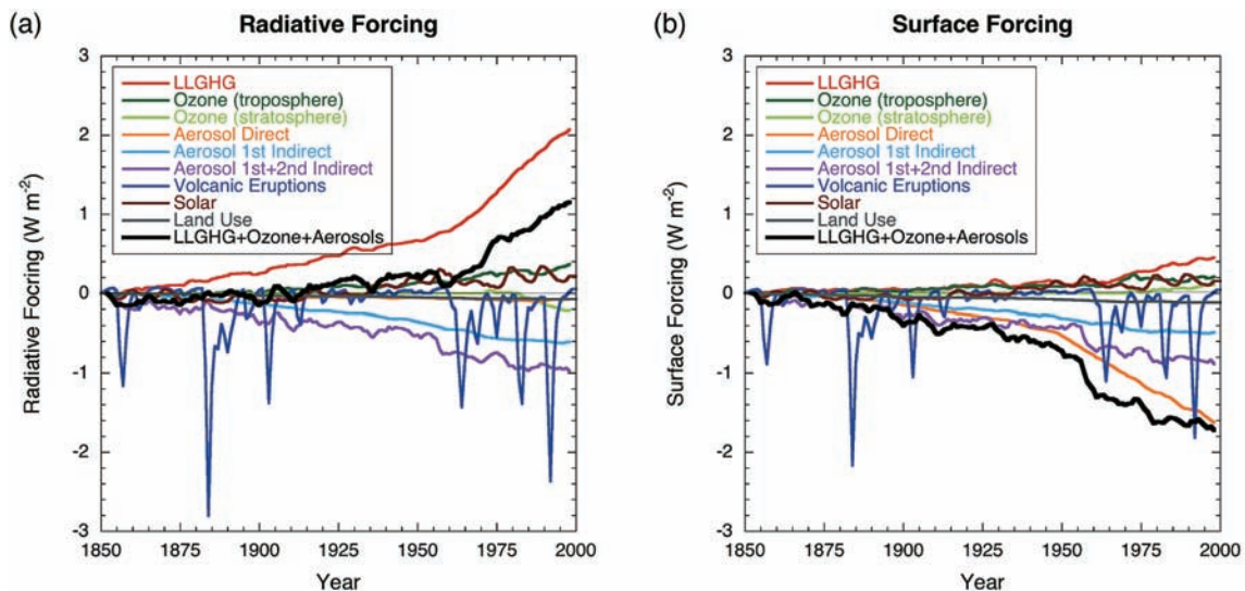
図1：(a)対流圏界面、(b)地表面における様々な気候強制因子による全天大気での1850～2000年の全球平均瞬時放射強制力の経年変化 (Takemura et al., 2006)．成層圏火山起源エアロゾル以外は5年移動平均を示す。
