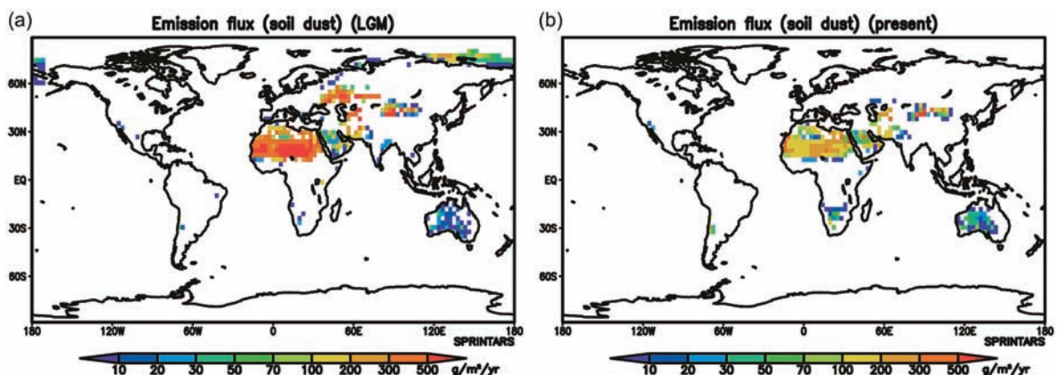
図2：(a)LGM、(b)現在気候における年間合計ダスト発生フラックスの全球分布 (Takemura et al., 2009)。
