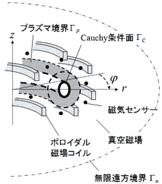
図1 Cauchy 条件面の配置
