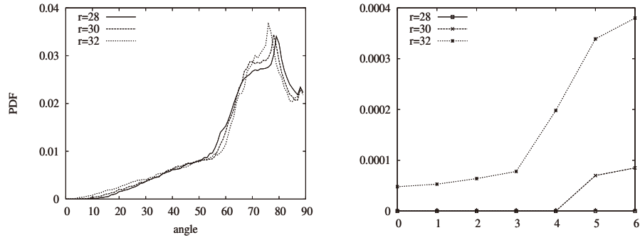
図 2: カオスアトラクタ上で安定多様体と不安定多様体のなすアングル出現頻度分布 ( r = 28, 30, 32 )(左)と詳細図(右) ( r を 28 から 32 に上げると小アングルの比率が増加し, r = 32 では 0 度付近に値をもつようになる)
