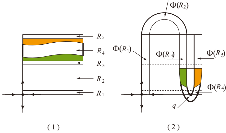
図 1.2: Cao-Luzzatto-Rios が用いたホモクリニック接触 q をもつ微分同相写像 \Phi .
