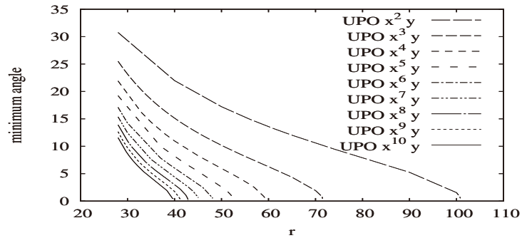
図 4: r を 28 から大きくしてサドルノード分岐点まで追跡した \text{UPO } x^N y^1 (グラフは上から順に N=2, 3, \dots, 10 ) の安定多様体と不安定多様体がなす最小アングル ( \text{UPO } x^N y^1 の最小アングル順は保存されるながら 0 に近づいていく様に見えるが, 実際には 0 には届かず正值に留まる)
