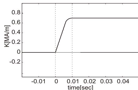
図 5: 渦電流時間変化
