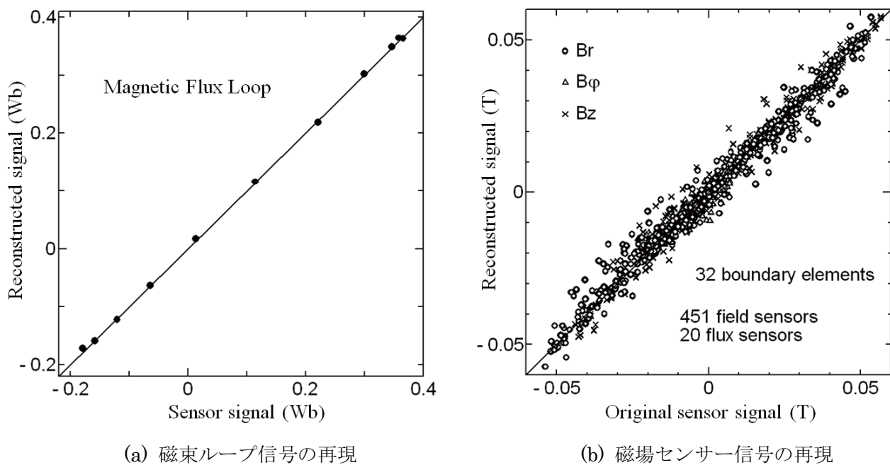
図2 LHD に対する計算結果
