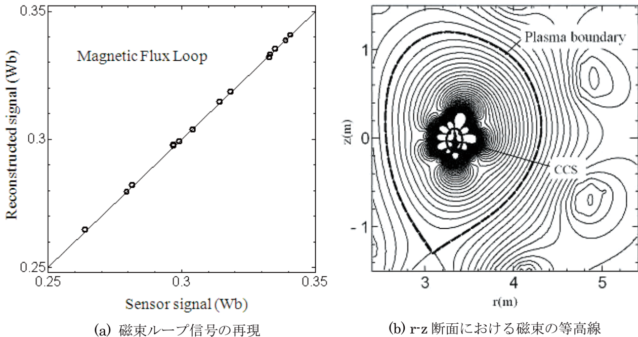
図1 JT-60 に対する計算結果
