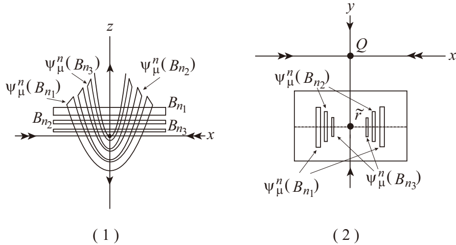
図 3.3: 定理 B の証明の概略．
