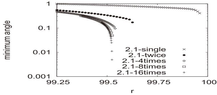
図 7: x^2y^1 ノード周期軌道の周期倍分岐周期軌道 (1, 2, 4, 8, 16 倍) の最小アングル
