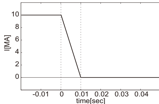
図 3: 強制入力したプラズマ電流の総和
