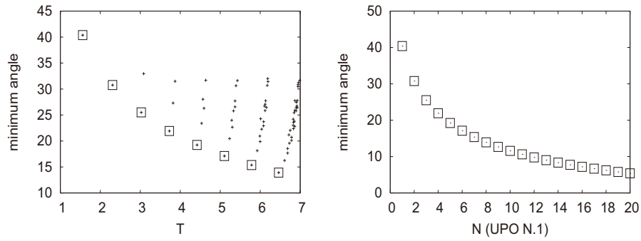
図 3: ポアンカレ写像周期 9 以下の各 UPO ( r = 28 )(左), \text{UPO } x^N y^1 ( N = 1, \dots, 20 )(右) 上で安定多様体と不安定多様体がなす最小アングル
