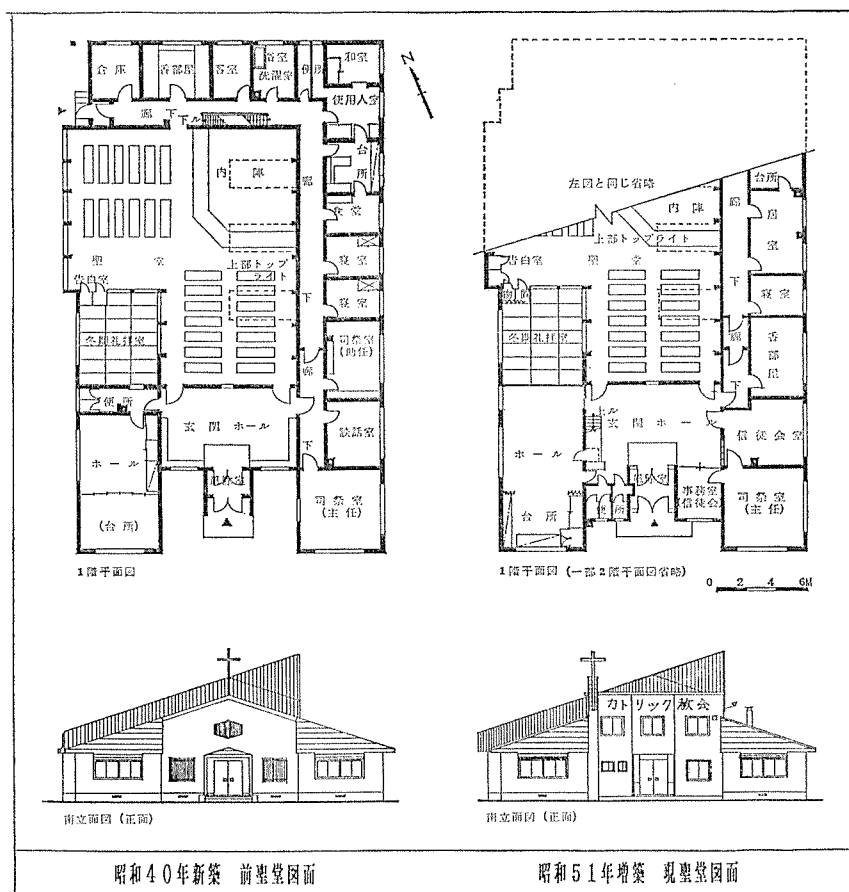
図一3 日本カトリック教会旭川大町教会 教会建築平面・立面変遷 復元・実測図 (2) (昭和40年～平成2年)
