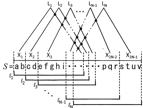
\ell_i は、辺のラベルが指し示す文字列の範囲を表す。図中の交点●の位置で新たな変数割当が必要となる。
