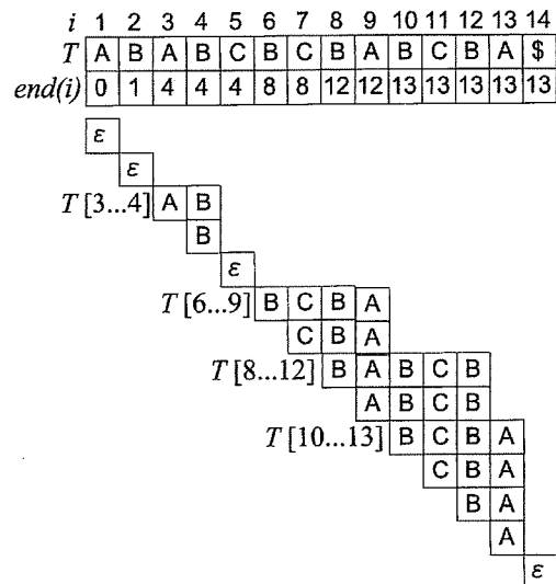
図 3 終了位置の配列 \text{end}(\cdot) と \text{Suf}(T, \pi) の関係
