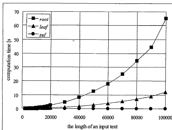
図 15 実験結果 3: T=AAA \cdots A\$ に対する実行時間の測定
