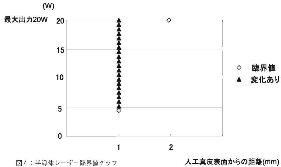
図4：半導体レーザー臨界値グラフ
