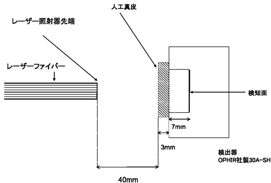
図2：人工真皮透過率の測定
