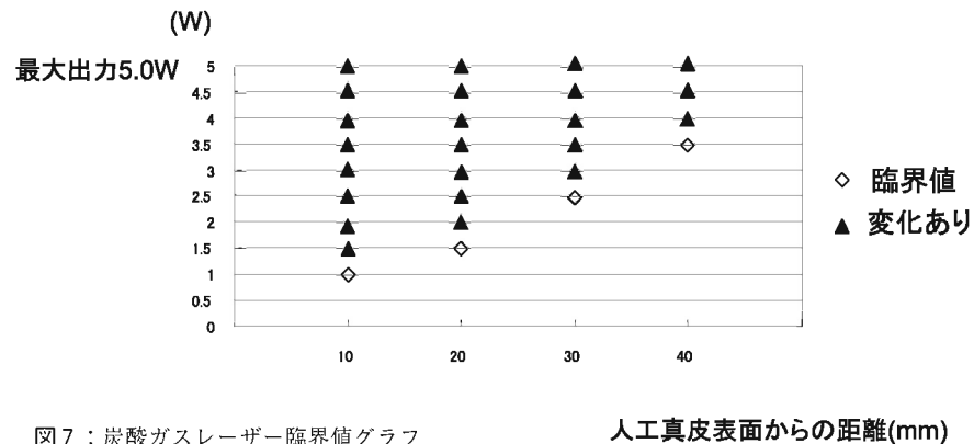
図7：炭酸ガスレーザー臨界値グラフ
