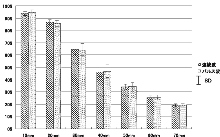
図 8：レーザー照射器先端と検知面の距離によるレーザー強度の差異
