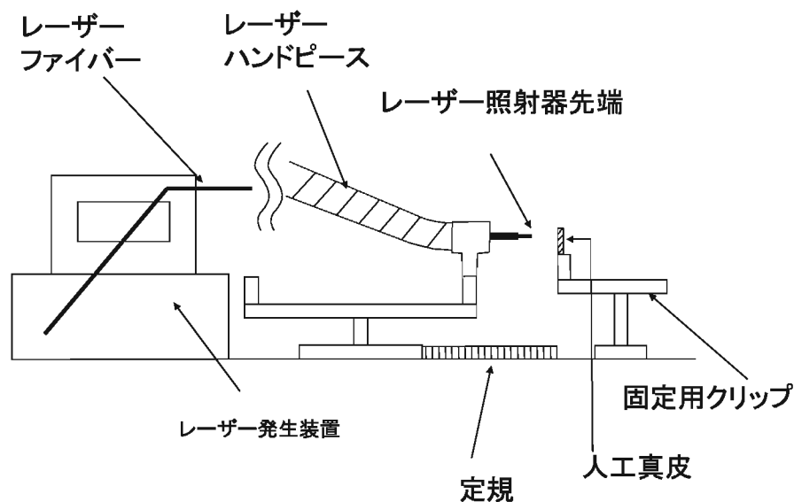
図 1：臨界値の測定模式図
