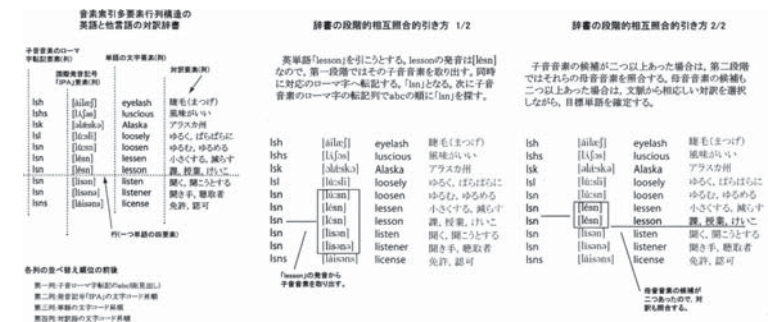
【図1】音素索引多要素行列構造の英語と他言語の対訳辞書とその段階的相互照合的引く方法の発明
