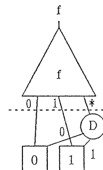
図 12 D 変数を最下位に置いた例 Fig. 12 D -variable in the lowest order.
