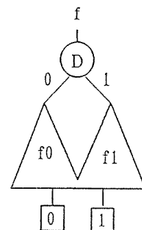
図 11 D 変数 Fig. 11 D -variable.
