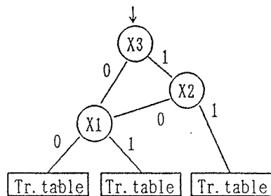
図 7 真理値表の併用
