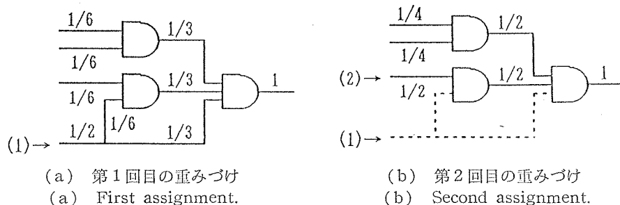
図9 動的重みづけ法
