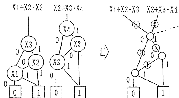
図 6 変数シフトエッジ Fig. 6 Variable shifters.
