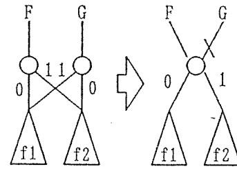
図 4 入力反転エッジ Fig. 4 Input inverters.
