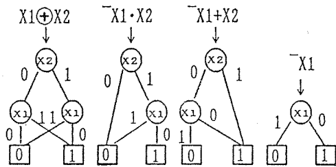
図 1 二分決定グラフ Fig. 1 BDD's.
