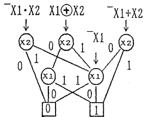
図 2 共有二分決定グラフ Fig. 2 SBDD.
