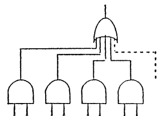
図 8 AND-OR 2段回路
