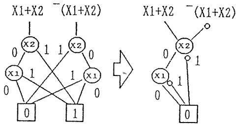
図 3 否定エッジ Fig. 3 Output inverters.
