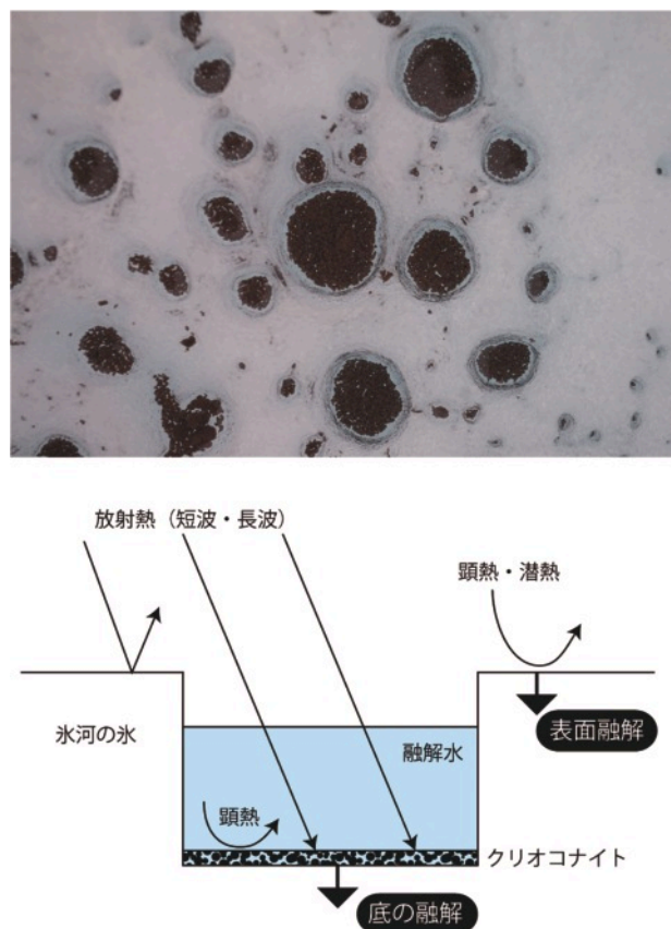
図6：クリオコナイトホール (Longyearbreen Glacier, Svalbard, 2011.8.21) とその形成過程。
