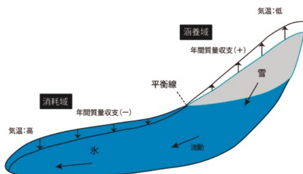
図 2: 氷河の断面図と標高による質量収支の違い。
