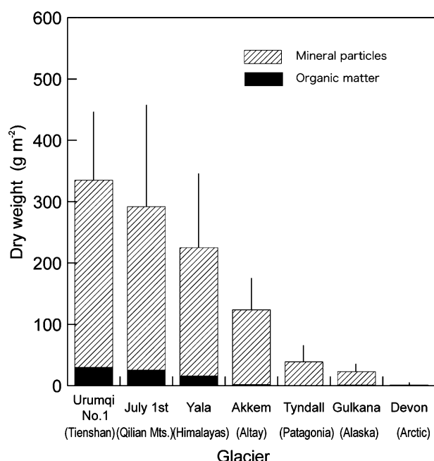
図8：消耗域の面積当たりのクリオコナイトの量（乾燥重量）の氷河間の比較。鉱物粒子と有機物のそれぞれの重量も示した。（Takeuchi and Li, 2008）
