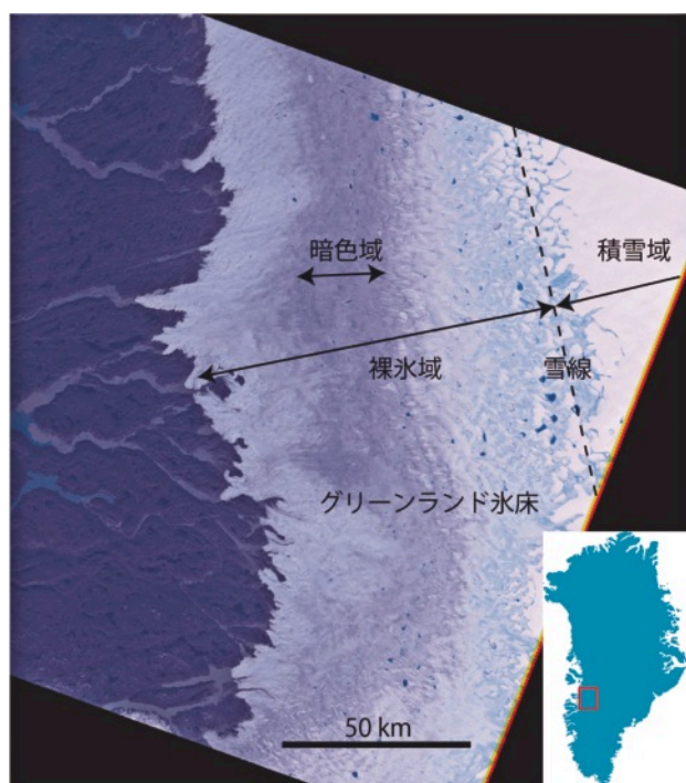
図 1: グリーンランド氷床西部の衛星写真。裸氷域に現れた暗色域を示した。(Landsat7 ETM+, Band1, 2, 3, 2000.8.23)
