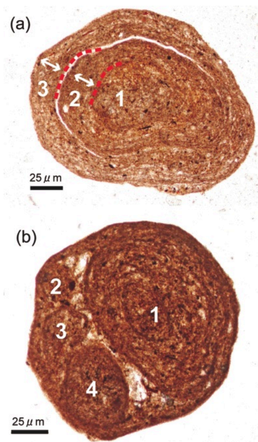
図5：クリオコナイト粒の断面の薄片写真。(a) 同心円の層構造、(b)複数の粒を内部に含む構造。(中国ウラムチ No.1 氷河のクリオコナイト粒, Takeuchi et al., 2010)
