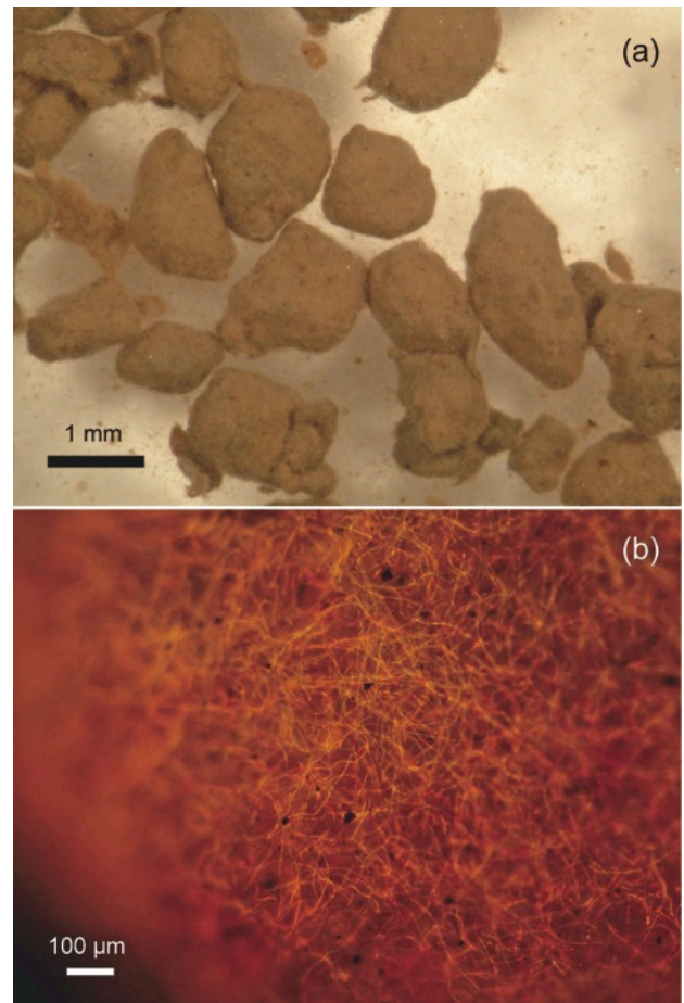
図 3：クリオコナイト粒の写真(a)と蛍光顕微鏡によるクリオコナイト粒の表面の写真(b)。オレンジに光るのは糸状のシアノバクテリア (中国ウルムチ No.1 氷河のクリオコナイト粒, Takeuchi et al., 2010)
