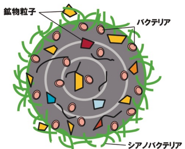
図 4：クリオコナイト粒の断面の模式図。ただし、バクテリア等の数や大きさは、見やすくするために変えているので本来ものと異なる。
