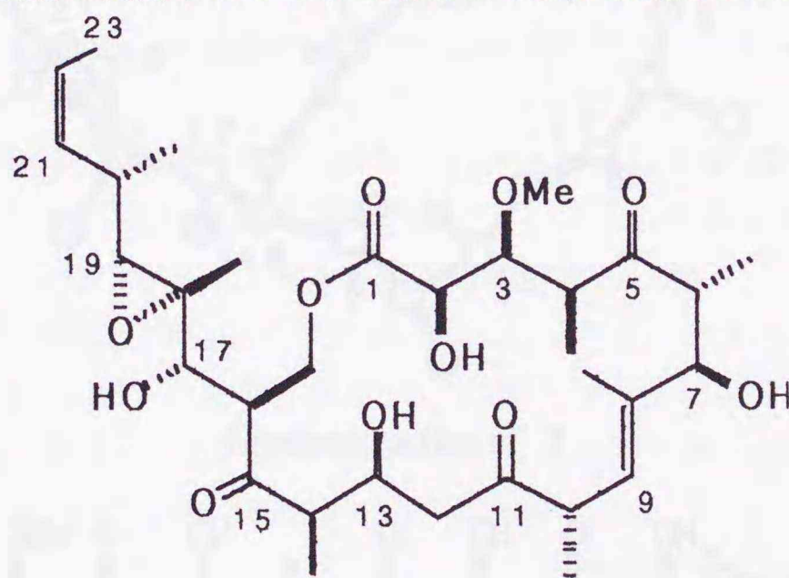
Tedanolide (1)
