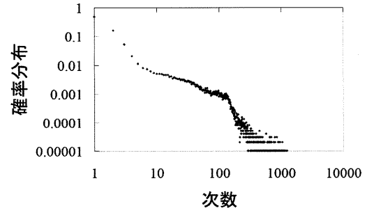
図 3: \mu = 0.9 における度数分布
