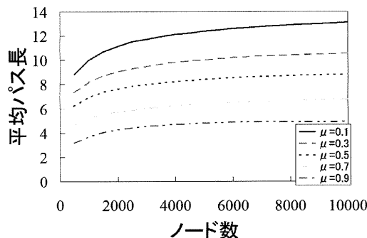
図 2: パス長の推移
