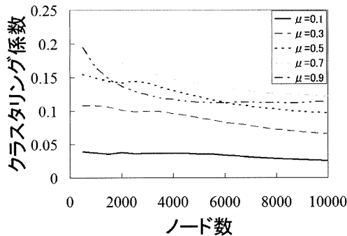
図 1: クラスタリング係数の推移
