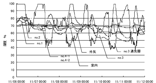
図4.4 2001/11/08-2001/11/12 壁体内湿度と外気湿度
