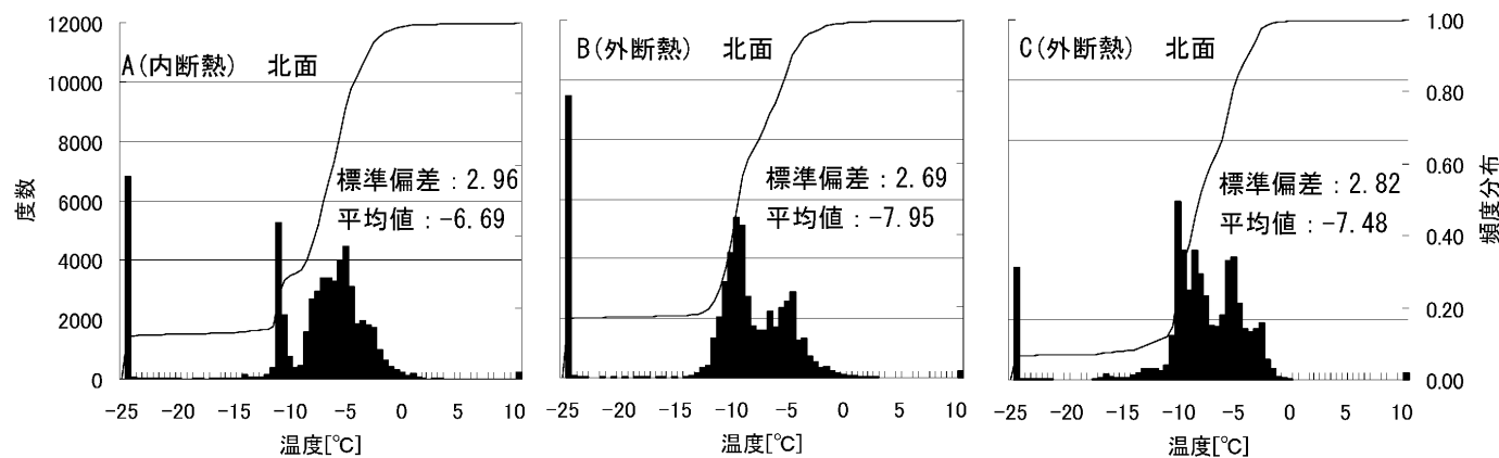
図4 北面の温度の頻度分布
