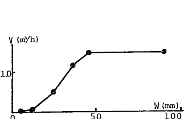
図7 中央高さ通過流量と中空層幅の関係
