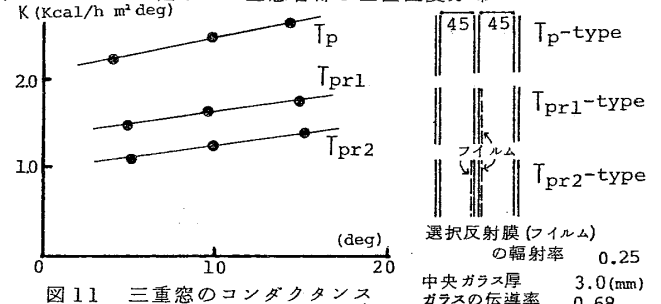
図11 三重窓のコンダクタンス
