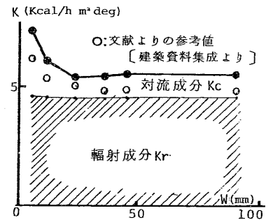
図6 コンダクタンスと中空層幅の関係
