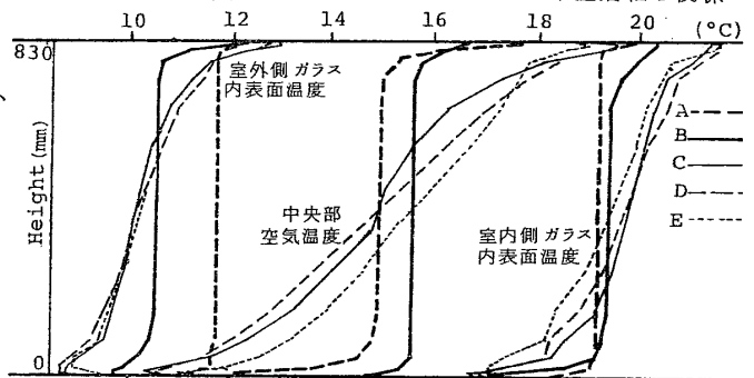
図9 二重窓各部の垂直温度分布
