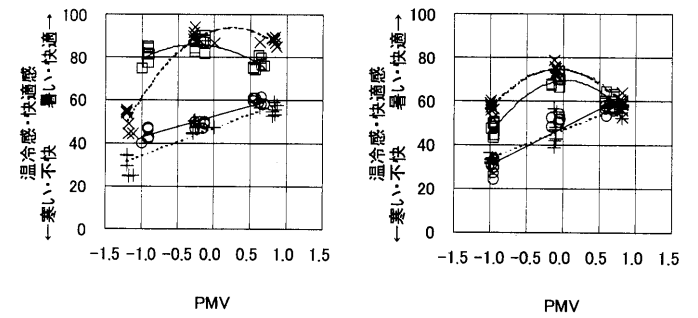
図10(a) PMVと心理反応(男性) 図10(b) PMVと心理反応(女性)
