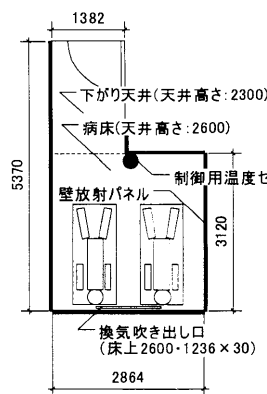
図1 人工気候室平面図 (単位・mm)
