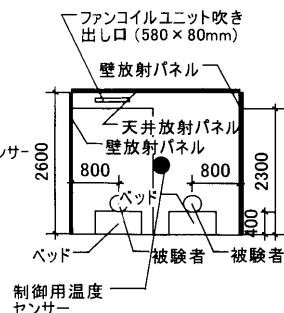
図2 人工気候室断面図 (単位・mm)
