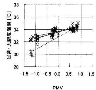
○—放射・足背 □—放射・大腿 ...+...対流・足背 ...×...対流・大腿 図8(a) PMVと生理反応 (男性)
