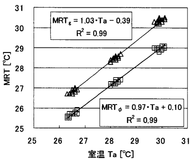
□MRTφ, △MRTg 図4 MRTφとMRTg
