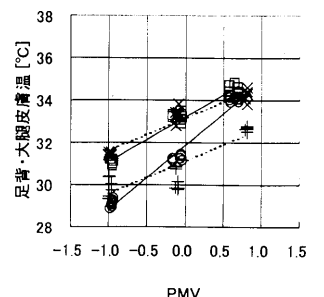
○—放射・足背 □—放射・大腿 ...+...対流・足背 ...×...対流・大腿 図8(b) PMVと生理反応 (女性)
