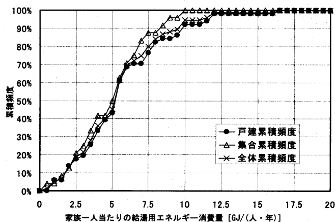
図 20 家族一人当たりの給湯用エネルギー消費量の割合の累積頻度
