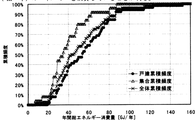
図9 年間総エネルギー消費量の累積頻度
