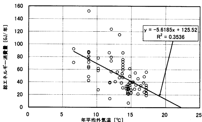
図14 年平均外気温と総エネルギー消費量の関係
