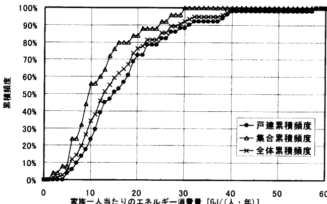
図13 家族一人当たりのエネルギー消費量の累積頻度
