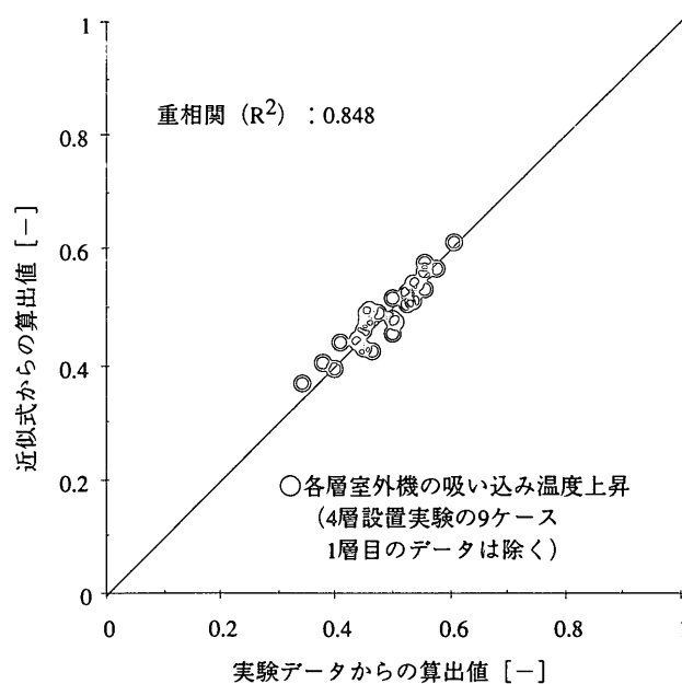
図14 外気流入率 R_m の実験値と計算値
