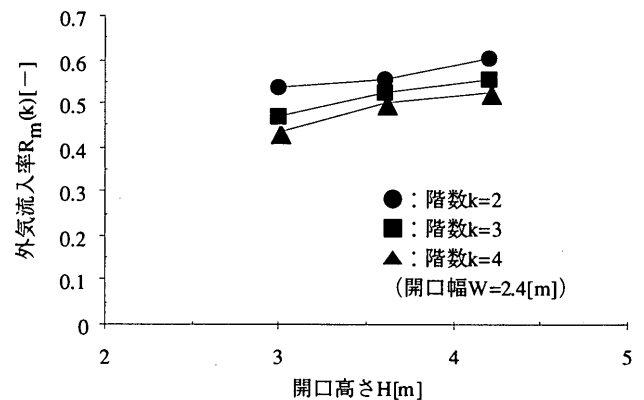
図13 開口高さHと外気流入率 R_m
