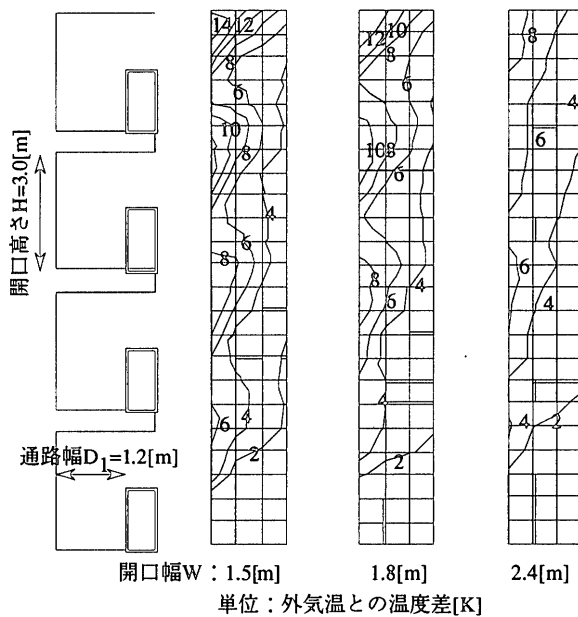
図10 バルコニー前面の空間温度分布
