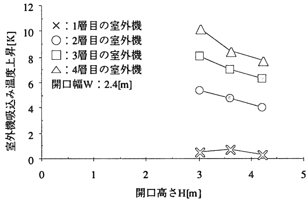
図9 開口高さHと吸込み温度上昇
