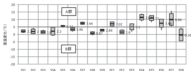
図6 住宅別の室温変化「入浴前・脱衣室」→「入浴後・居間」
