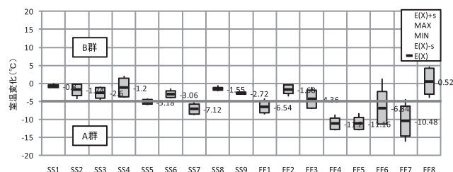
図5 住宅別の室温変化「入浴前・居間」→「入浴前・脱衣室」
