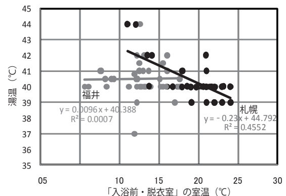
図 4 札幌と福井の脱衣室の室温に対する湯温
