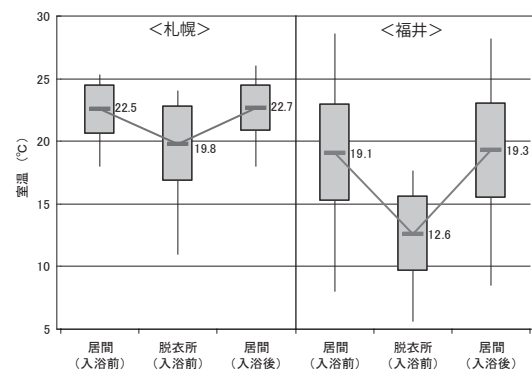
図 3 札幌と福井の居間と脱衣室の室温変化
