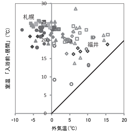
図 1 外気温と「入浴前・居間」の室温
