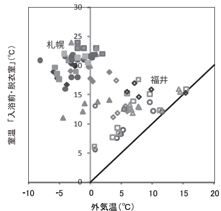
図 2 外気温と「入浴前・脱衣室」の室温
