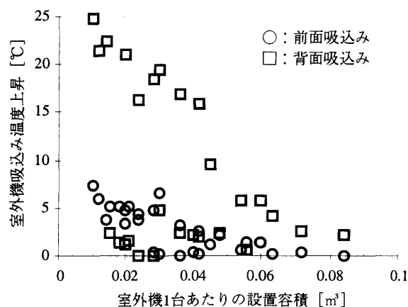
図6 1層設置での吸込み温度上昇
