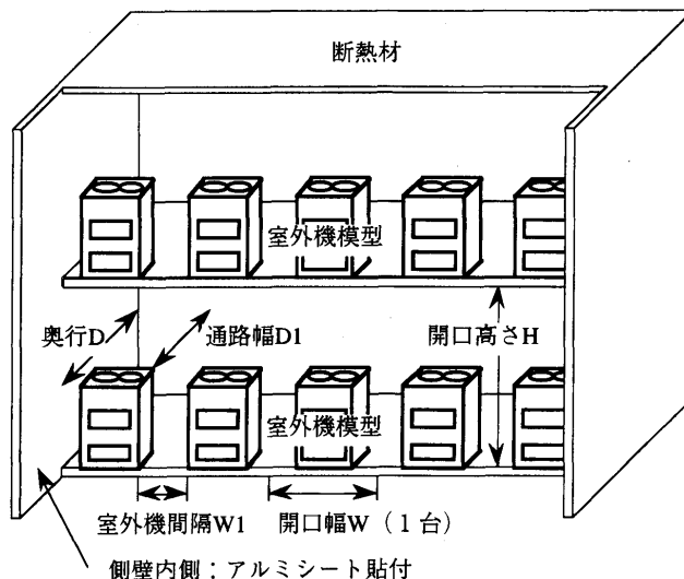
図5 室外機模型実験の概要
