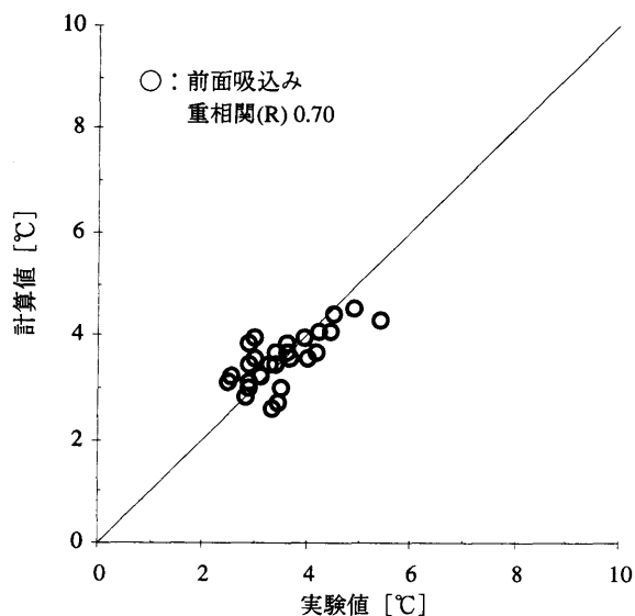
図10 吸込み温度上昇の実験値と計算値（2層設置）
