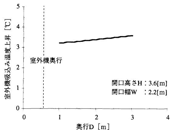
奥行Dと室外機吸込み温度上昇
