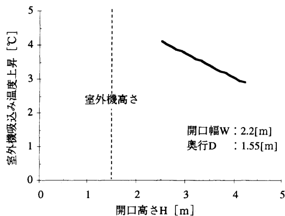
開口高さHと室外機吸込み温度上昇
