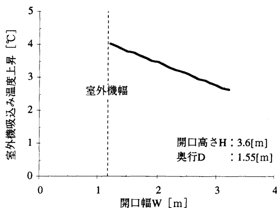
開口幅Wと室外機吸込み温度上昇
