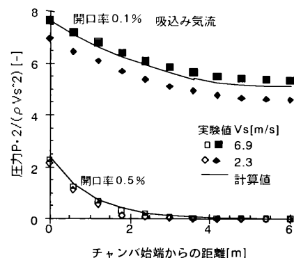
図7 吹出し・吸込み気流の実験と計算結果
