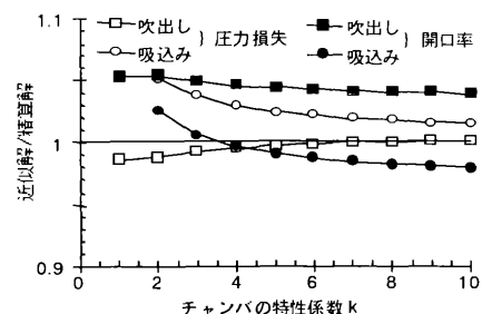
図5 近似式の精度 ( \varepsilon=0.3 )
