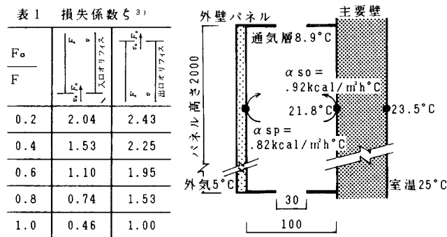
図4 計算結果例
