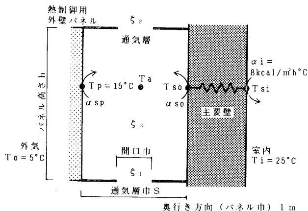
図3 伝熱モデル (立断面)
