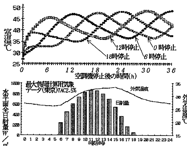
図2 空調システム停止後の室温変化の計算例
