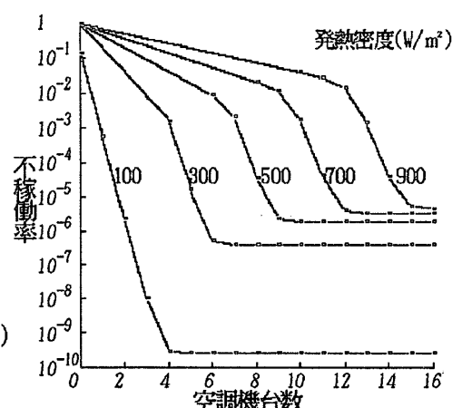
図4 空調システム不稼働率の計算例
