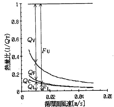
図4 循環面風速と熱収支の関係
