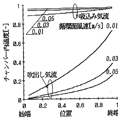
図2 循環面風速とチャンバー内温度の関係
