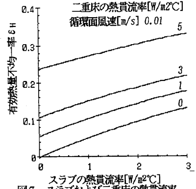
図7 スラブおよび二重床の熱貫流率と熱量の不均一率の関係
