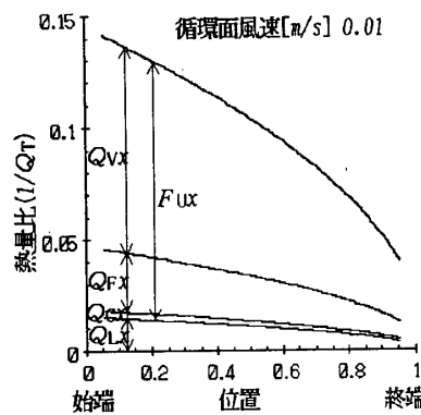
図3 各位置における熱収支
