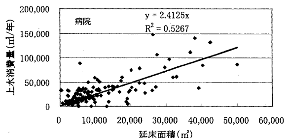
図 5 延床面積と上水消費量（病院）
