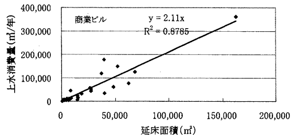
図 3 延床面積と上水消費量（商業ビル）
