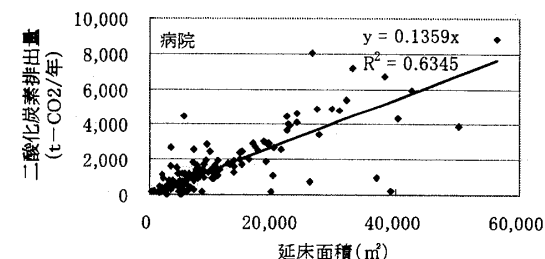
図11 延床面積とCO2排出量 (病院)
