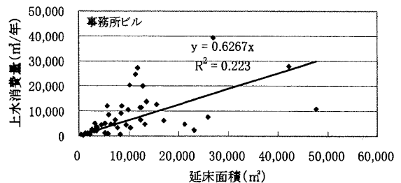
図 2 延床面積と上水消費量（事務所ビル）
