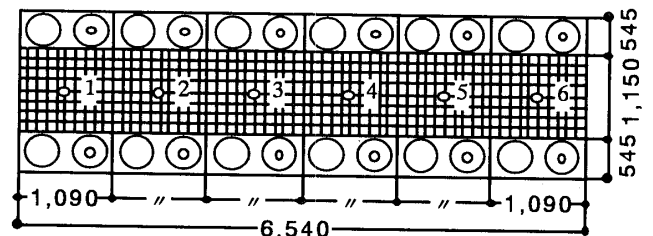
【平面配置図】
