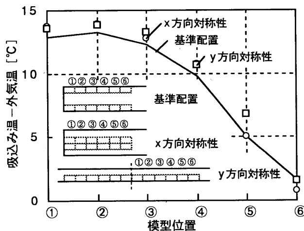
図-6 対称性実験結果比較
