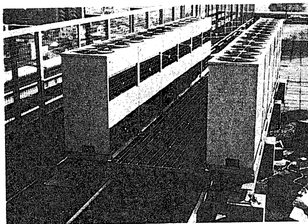
図-3 実測室外機の設置状況
