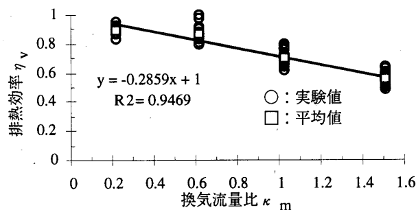
図2 排熱効率
