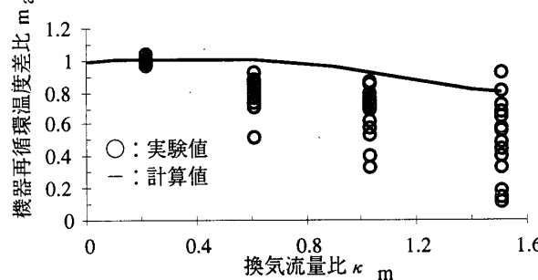
図5 機器再循環温度差比
