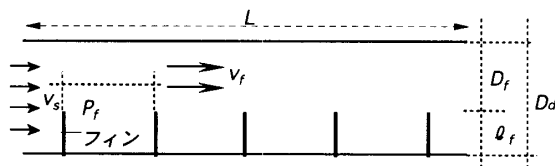
図3 フィン付きチャンバのモデル
