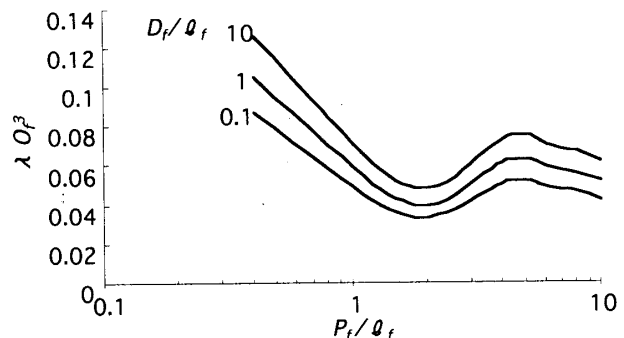
図5 フィン付きチャンバの通気抵抗
