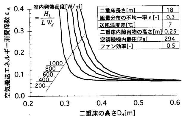
図6 二重床の高さと空気搬送エネルギー消費係数
