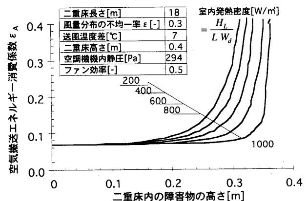
図7 二重床内の障害物高さと空気搬送エネルギー消費係数
