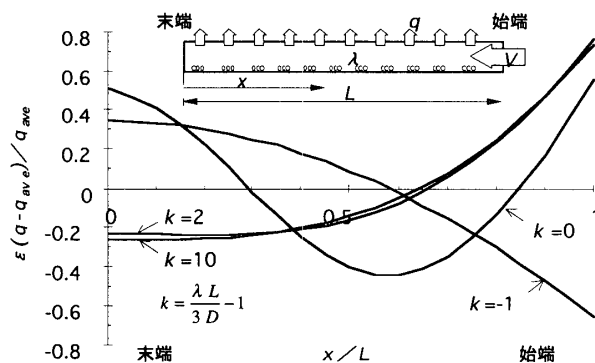
図1 吹出し風量分布
